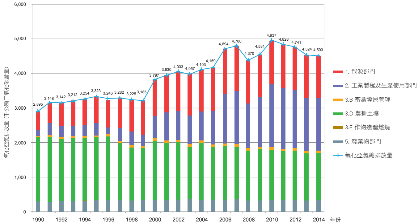
圖 2.2.3 臺灣 1990 至 2014 年氧化亞氮排放量趨勢
