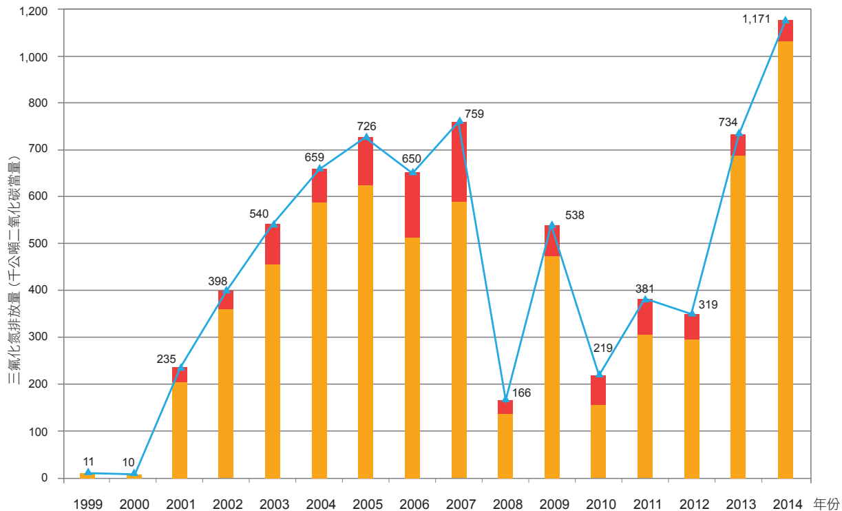
圖 2.2.7 臺灣 1999 至 2014 年三氟化氮排放量趨勢
