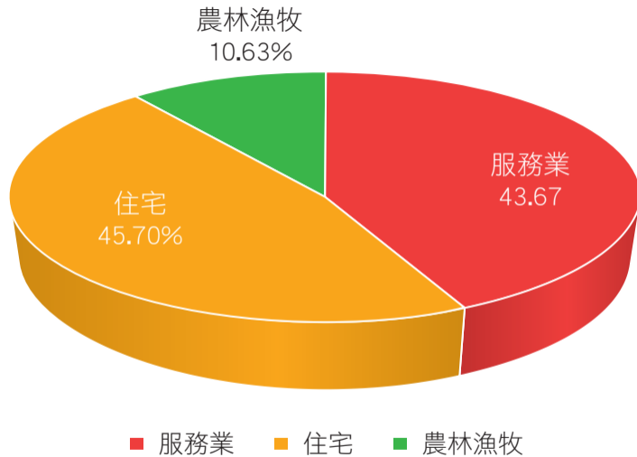
圖 3.2.27 臺灣 2014 年服務、住、農林漁牧部門燃料燃燒二氧化碳排放量占比
