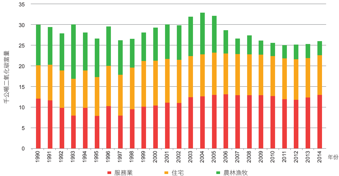
圖 3.2.28 臺灣 1990 至 2014 年服務、住、農林漁牧部門燃料燃燒甲烷排放量趨勢
