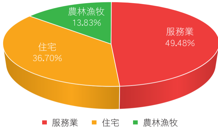
圖 3.2.29 臺灣 2014 年服務、住、農林漁牧部門燃料燃燒甲烷排放量占比
