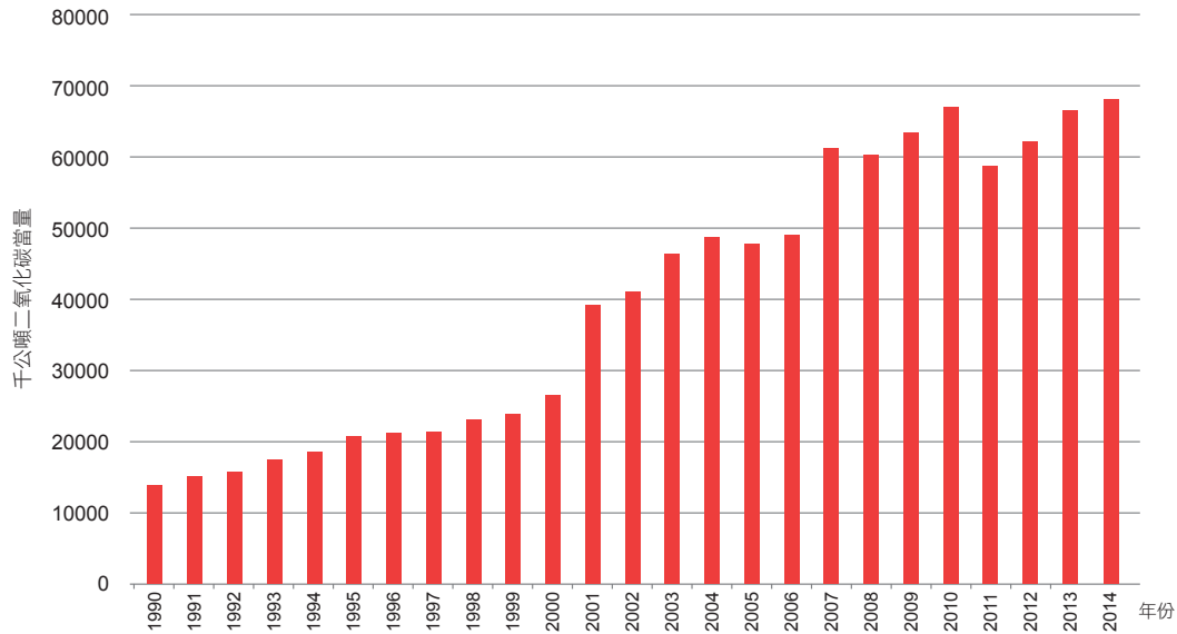
圖 3.2.38 臺灣 1990 至 2014 年非能源使用燃料燃燒二氧化碳扣減量趨勢
