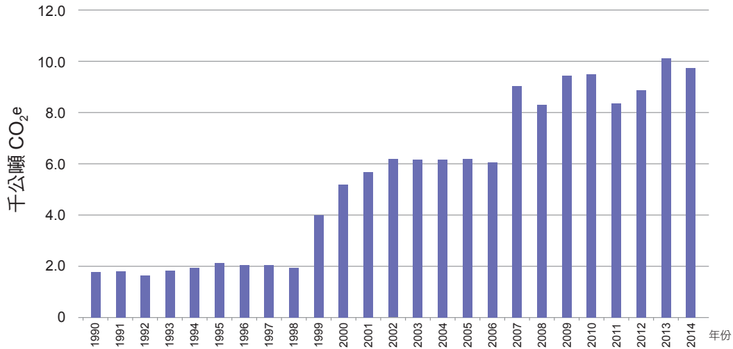
圖 4.3.15 臺灣 1990 至 2014 年苯乙烯生產排放量趨勢
