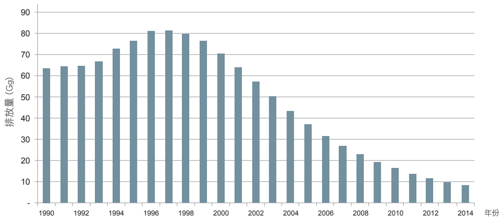
圖 7.2.2 臺灣 1990 至 2014 年未妥善管理廢棄物掩埋場甲烷排放量趨勢
