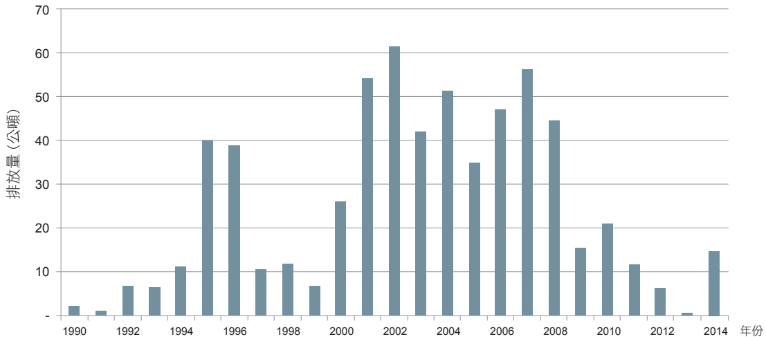
圖 7.4.2 臺灣 1990 至 2014 年廢棄物焚化二氧化碳排放量趨勢
