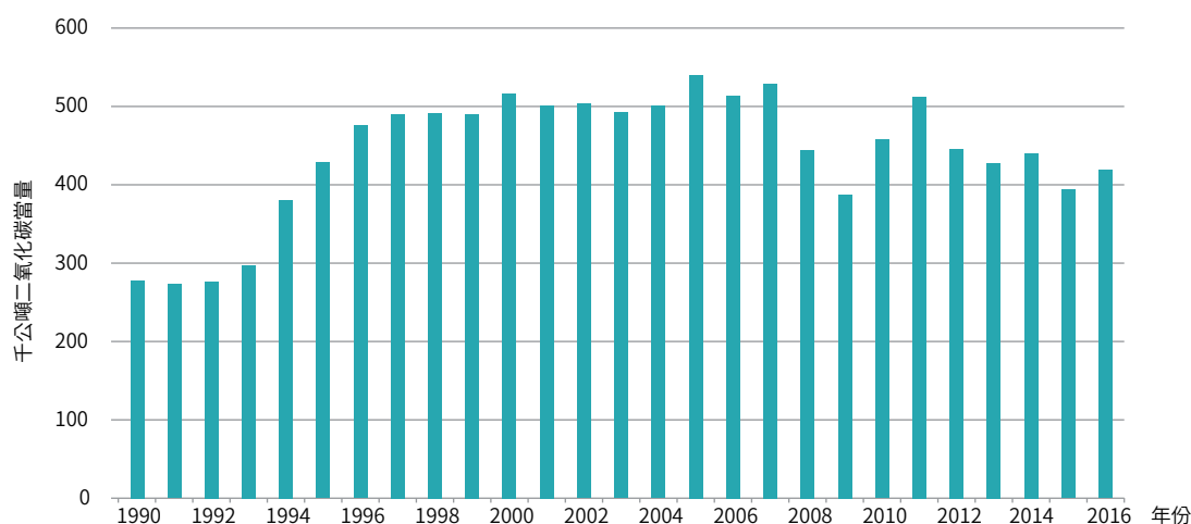
圖 4.3.13 臺灣 1990 至 2016 年碳黑生產排放量趨勢
