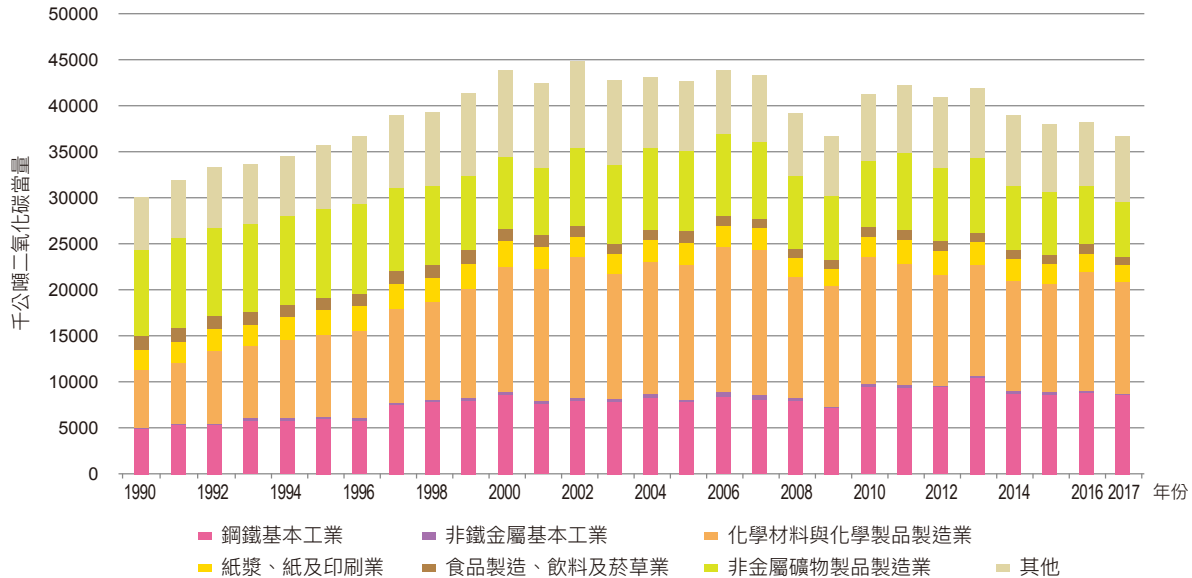
圖 3.2.14 臺灣 1990 至 2017 年製造業與營造業燃料燃燒二氧化碳排放趨勢
